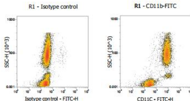
图. 人外周血染色, 左图为Rat IgG2a, κ Isotype control, FITC的结果, 右图为Anti-Human/Mouse CD11b, FITC的结果。以淋巴细胞、粒细胞和单核细胞设门进行分析
