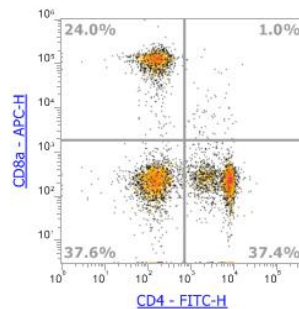
图. 大鼠抗凝血染色 Anti-Rat CD4, FITC (F3100401)和 Anti-Rat CD8α, APC (F3100803)的结果。 已排除黏连细胞。
