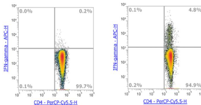
图. ICR 小鼠脾细胞经 PMA/Ionomycin (CS1001)刺激和 BFA/Monensin (CS1002)阻断后, 对生物学对照组(左)和实验组(右)染色 Anti-Mouse CD4, PerCP-Cy5.5 (F2100404)和 Anti-Mouse IFN- \gamma , APC (F21IFNG03)的结果。以 CD3+细胞设门分析。已排除黏连细胞。
