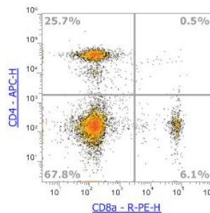
图. ICR 小鼠脾细胞染色 Anti-Mouse CD8 \alpha , PE (F21008A02)和 Anti-Mouse CD4, APC (F2100403)的结果。已排除粘连细胞。
