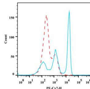
图. 人外周血染色 Anti-Human CD33, PE-Cyanine7 (F1103305)(实线)和 Mouse IgG1 κ Isotype Control, PE-Cyanine7(CMG104)(虚线)的结果。以 FSC/SSC 中的单核细胞设门进行分析。
