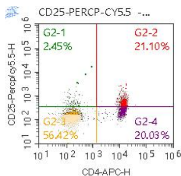
图. 人外周血染色 Anti-Human CD4, APC (F1100403)和Anti-Human CD25, PerCP-Cy5.5 (F1102504/2) 的结果。以 FSC/SSC 中的淋巴细胞设门进行分析。
