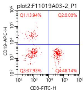
图. 人外周血染色 Anti-Human CD19, APC (F11019A03/2)和Anti-Human CD3, FITC (F11003A01)的结果。以 FSC/SSC 中的淋巴细胞设门进行分析。
